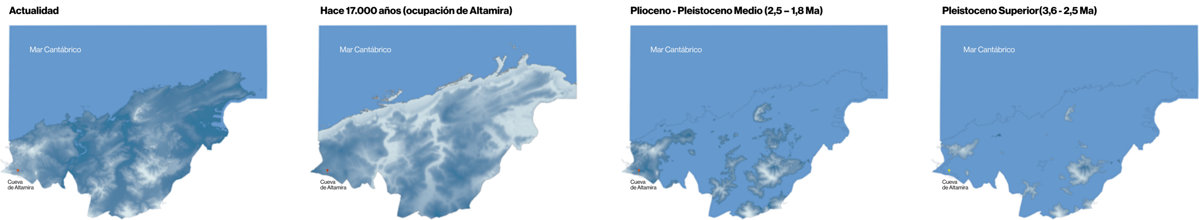
Figuras en las que se representan las tierras emergidas en los diferentes períodos geológicos. Los diferentes tonos de blanco y celeste se representa el Modelo Digital de Elevaciones de las tierras emergidas.
